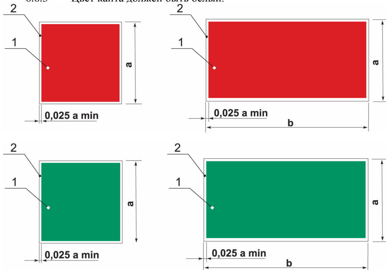
а, b – сторона квадрата и прямоугольника; 1 – основная поверхность; 2 – кант Рисунок 4 – Основа цветографического изображения и соотношение размеров указательных знаков пожарной безопасности
