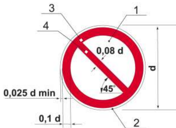
d – диаметр круга; 1 – основная поверхность; 2 – кант; 3 – кайма; 4 – поперечная полоса Рисунок 1 – Основа цветографического изображения и соотношение размеров
